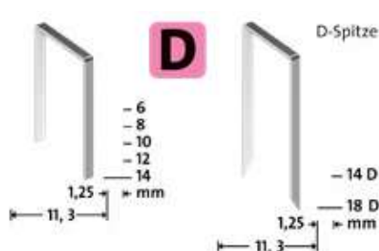
NOVUS Graffetta piatta D, Tipo 53F
